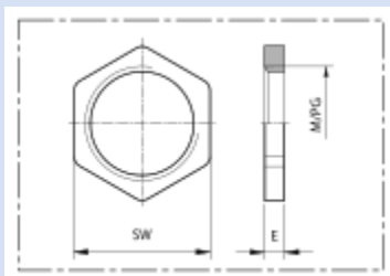
Kovová matka s protizávitem
